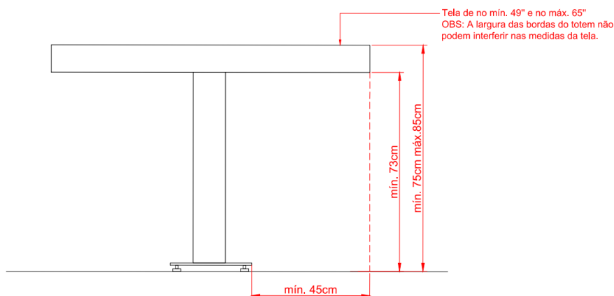
VISTA LATERAL TOTEM HORIZONTAL
